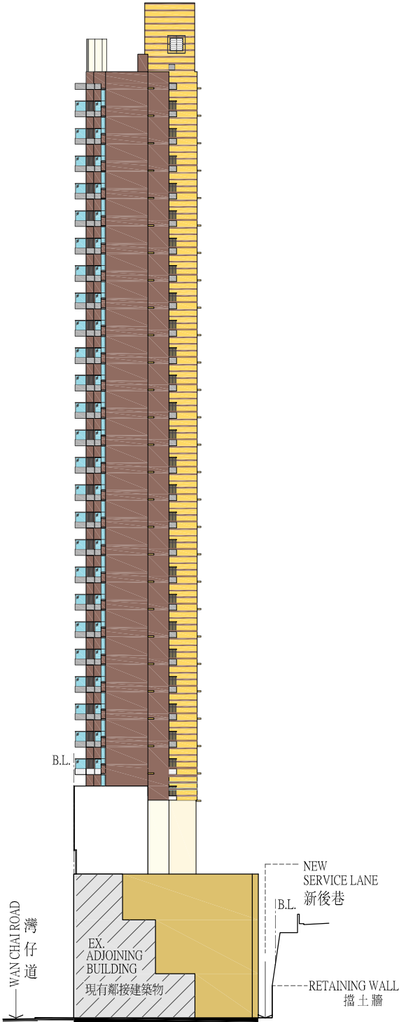
ELEVATION 3 - EX. BUILDING 立面圖 3 - 面向現有鄰接建築物
