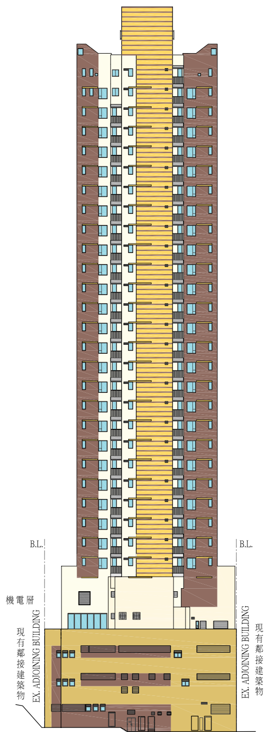
ELEVATION 2 - NEW SERVICE LANE 立面圖 2 - 面向新後巷
